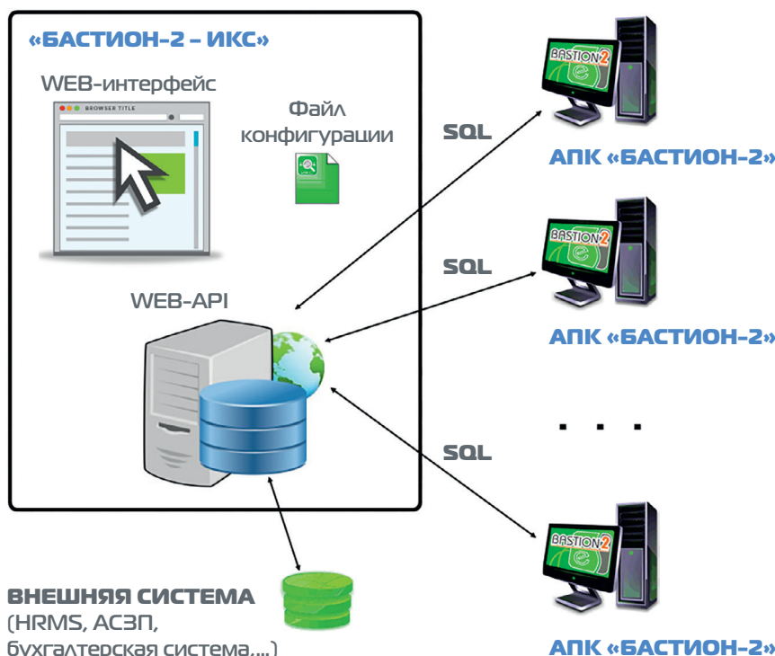
Рис. 1. Схема интеграции внешних систем с использованием «Бастион-2-ИКС»
