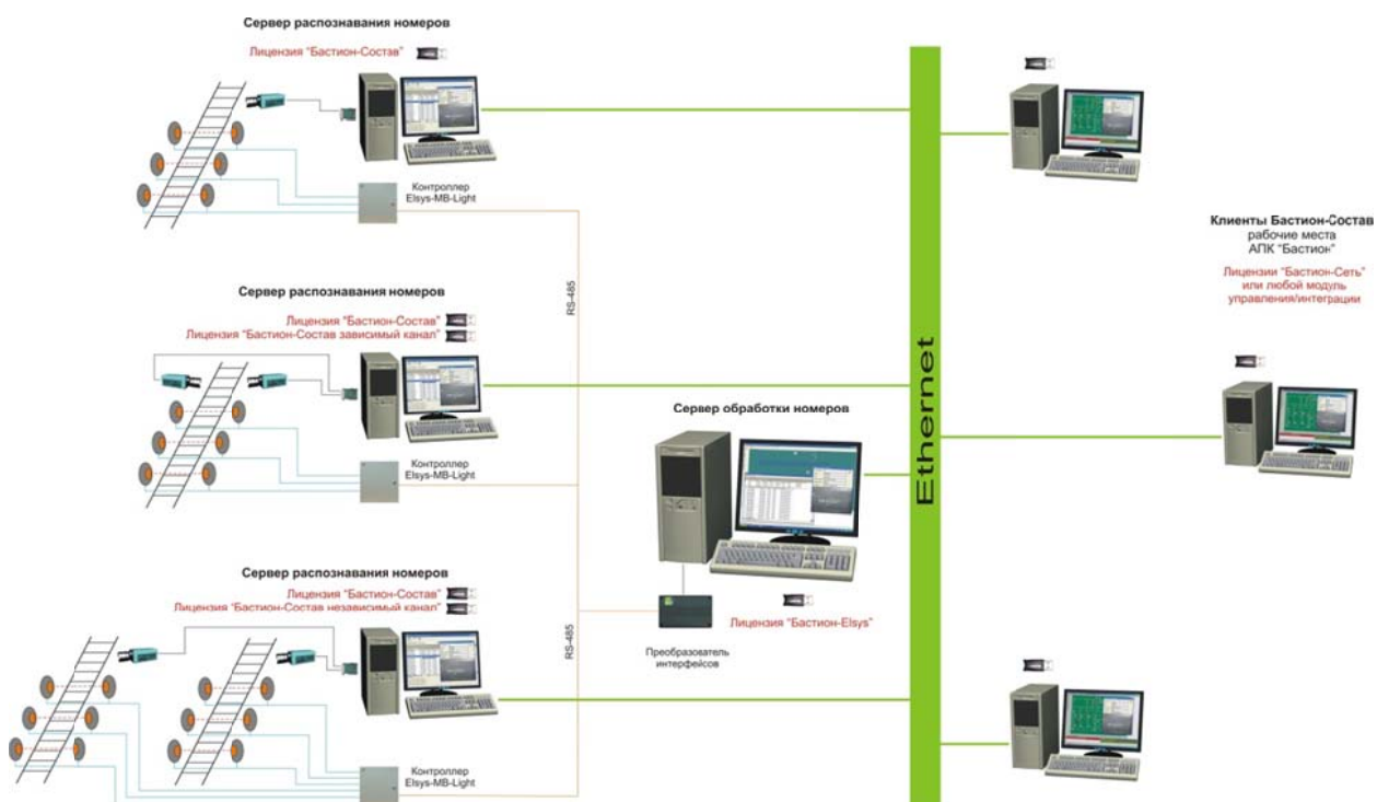
Рисунок 4 – Конфигурация «Бастион-Состав» с выделенными серверами распознавания и обработки номеров
