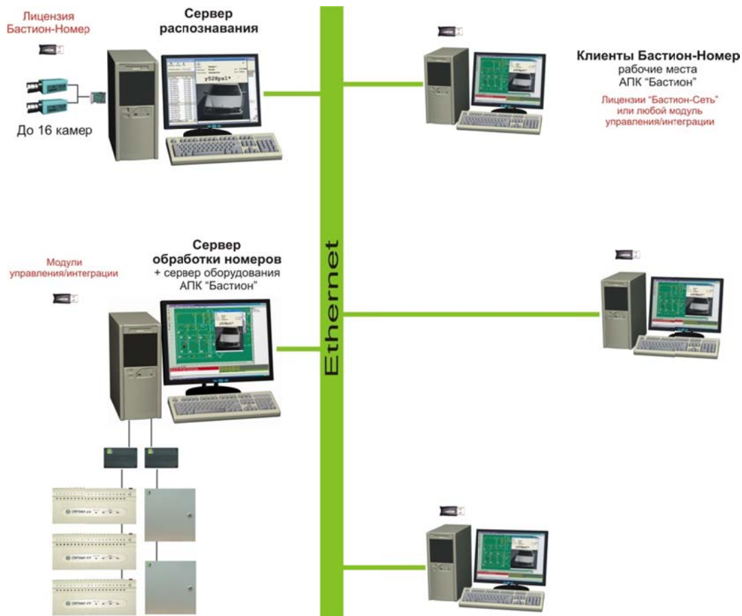
Рисунок 3 – «Бастион-Номер», сервер обработки номеров совмещен с сервером оборудования АПК «Бастион»
