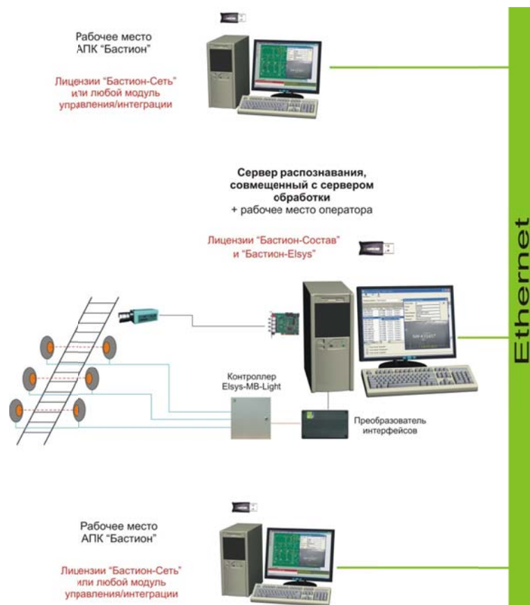
Рисунок 5 – Конфигурация «Бастيون-Состав», сервер распознавания и обработки на одном компьютере
