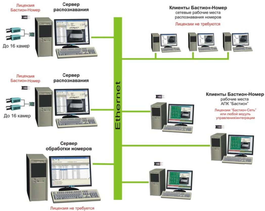
Рисунок 1 – Конфигурация «Бастион-Номер» с выделенными серверами распознавания и обработки
