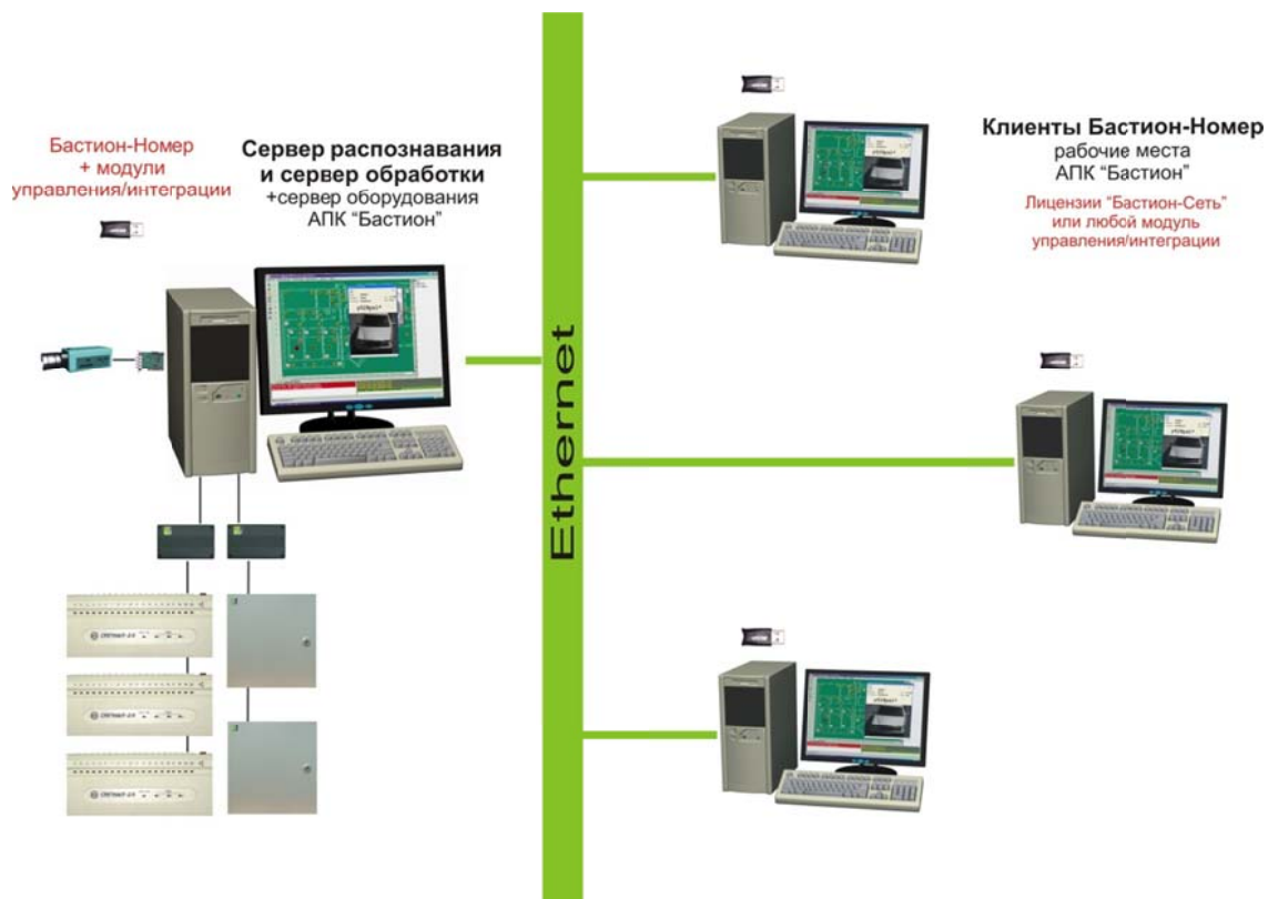
Рисунок 2 – «Бастион-Номер», полностью реализованный на одном компьютере совместно с сервером оборудования АПК «Бастион»
