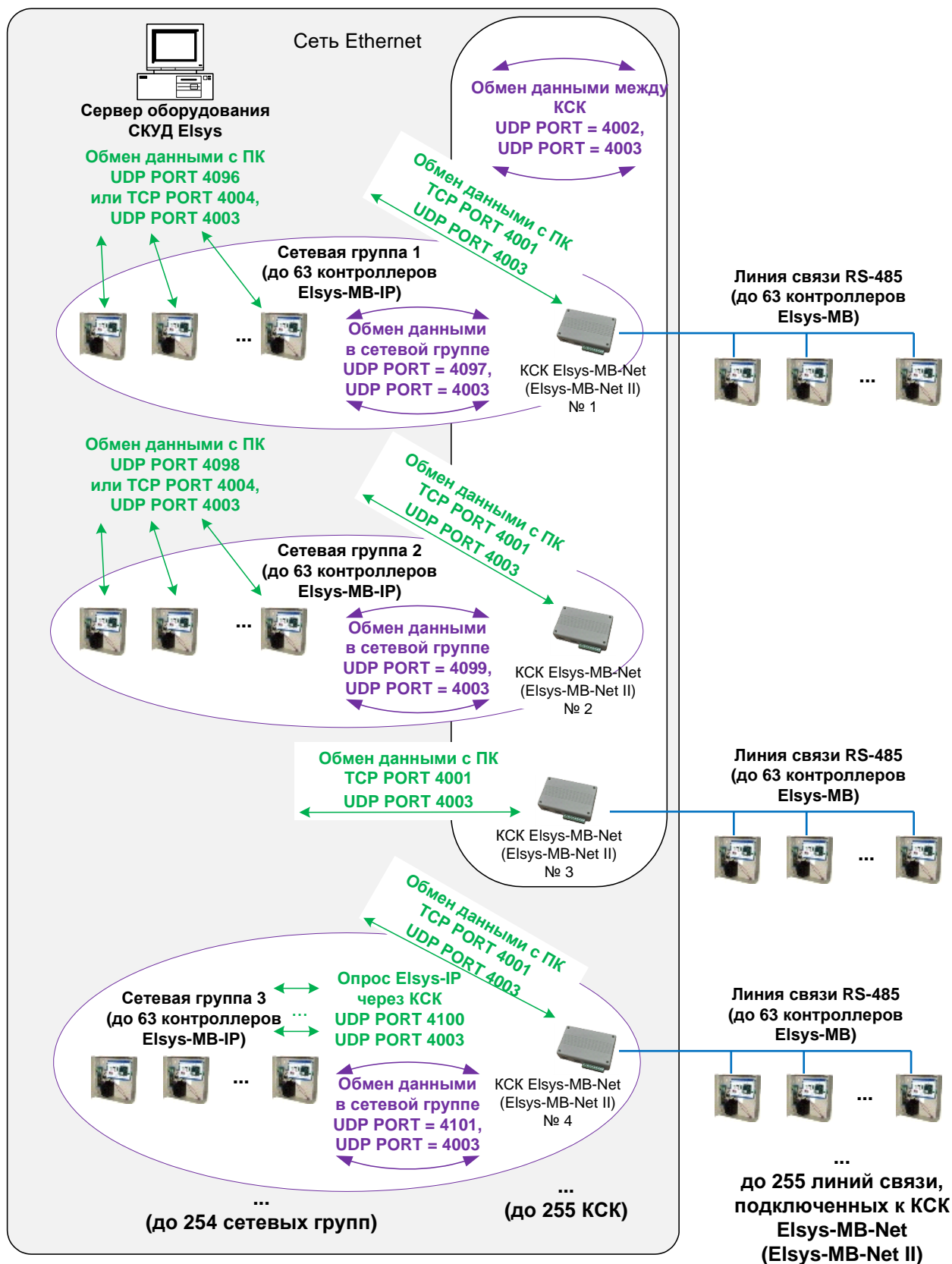
Рисунок 1 – Использование КСК Elsys-MB-Net II в составе СКУД Elsys
